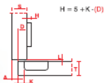
Polkriva spona, C = 9
