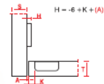
Kriva spona, C = 18
